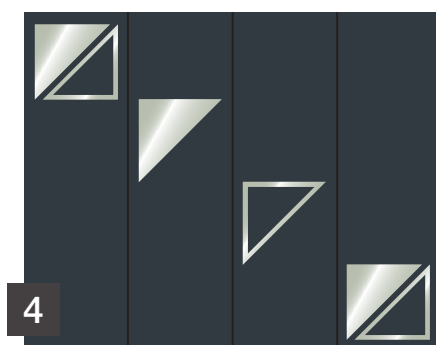
Modèle 4 : • 3 motifs triangles : 400 x 400 mm • 3 motifs triangles évidés : 400 x 400 mm
