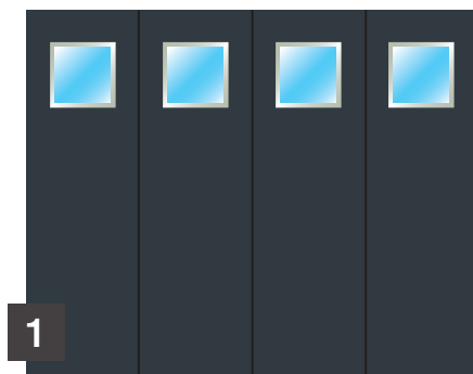
Modèle 1 : • 4 hublots collés ABA carrés vitrage composite glace PMMA sablé : 300 x 300 mm
